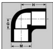
90° ELL (Slip x Slip)
